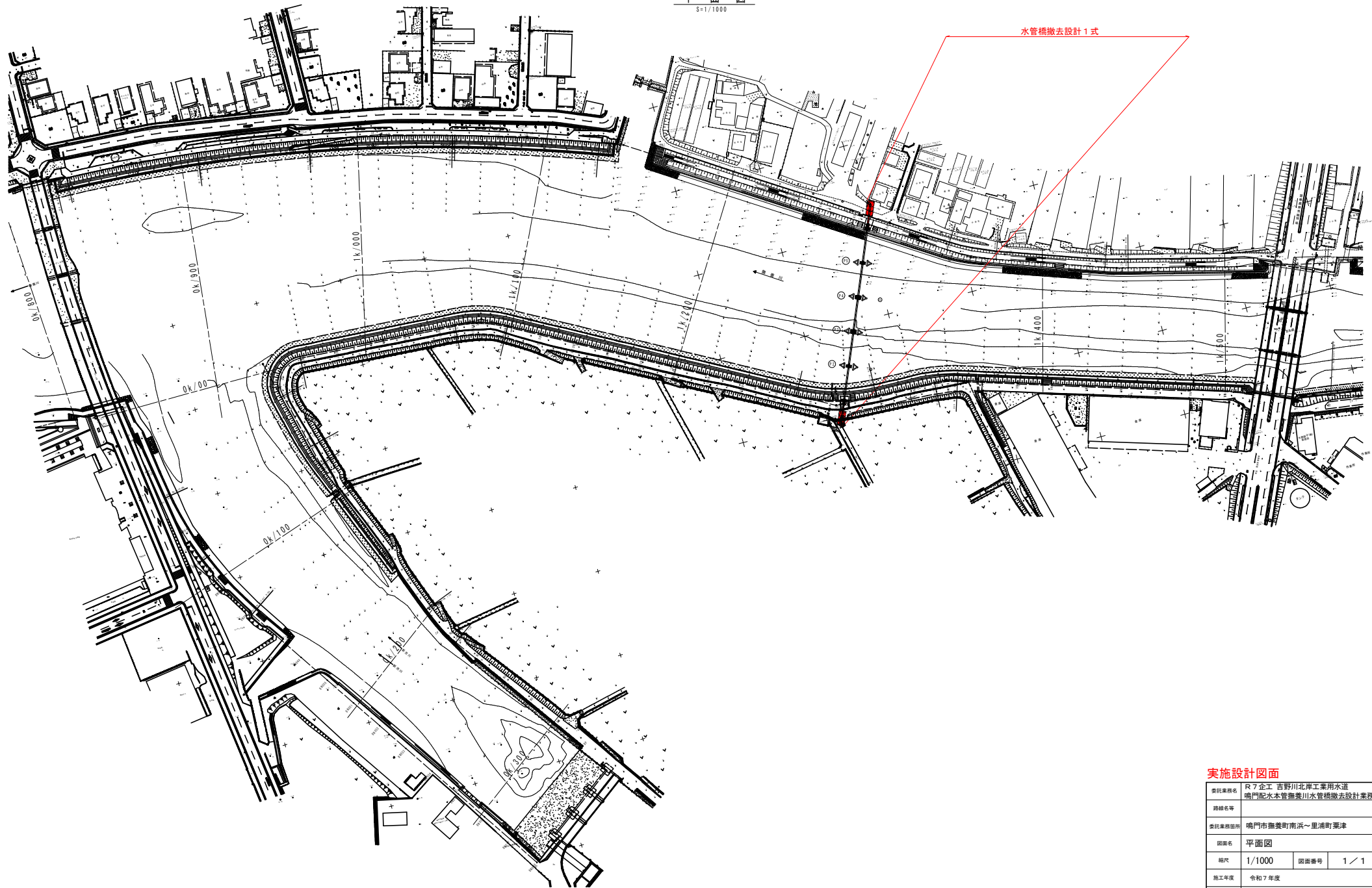
平面図 S=1/1000
